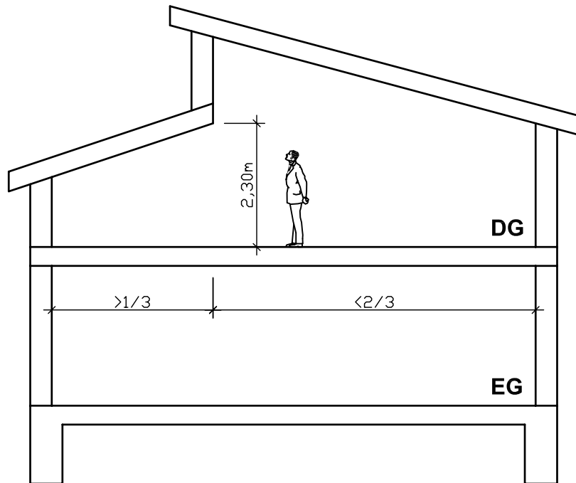
Standard-Vorschlag 1 für ein nicht anzurechnendes Dachgeschoss geringer Dachneigung nach novellierter LBauO M-V
