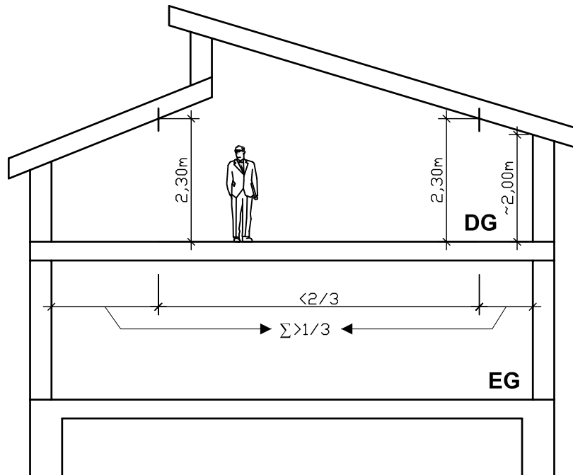
Standard-Vorschlag 2 für ein nicht anzurechnendes Dachgeschoss geringer Dachneigung nach novellierter LBauO M-V
